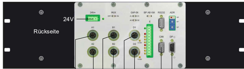
Auswuchtelektronik 3.AB340P01.C.KM.V2AA.DPV1
